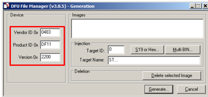
Рисунок 55. Область Device
