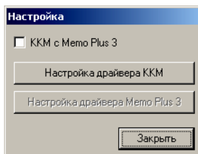
Рисунок 36. Окно «Настройка»
